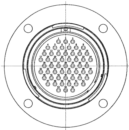
セン受正面(55芯)
